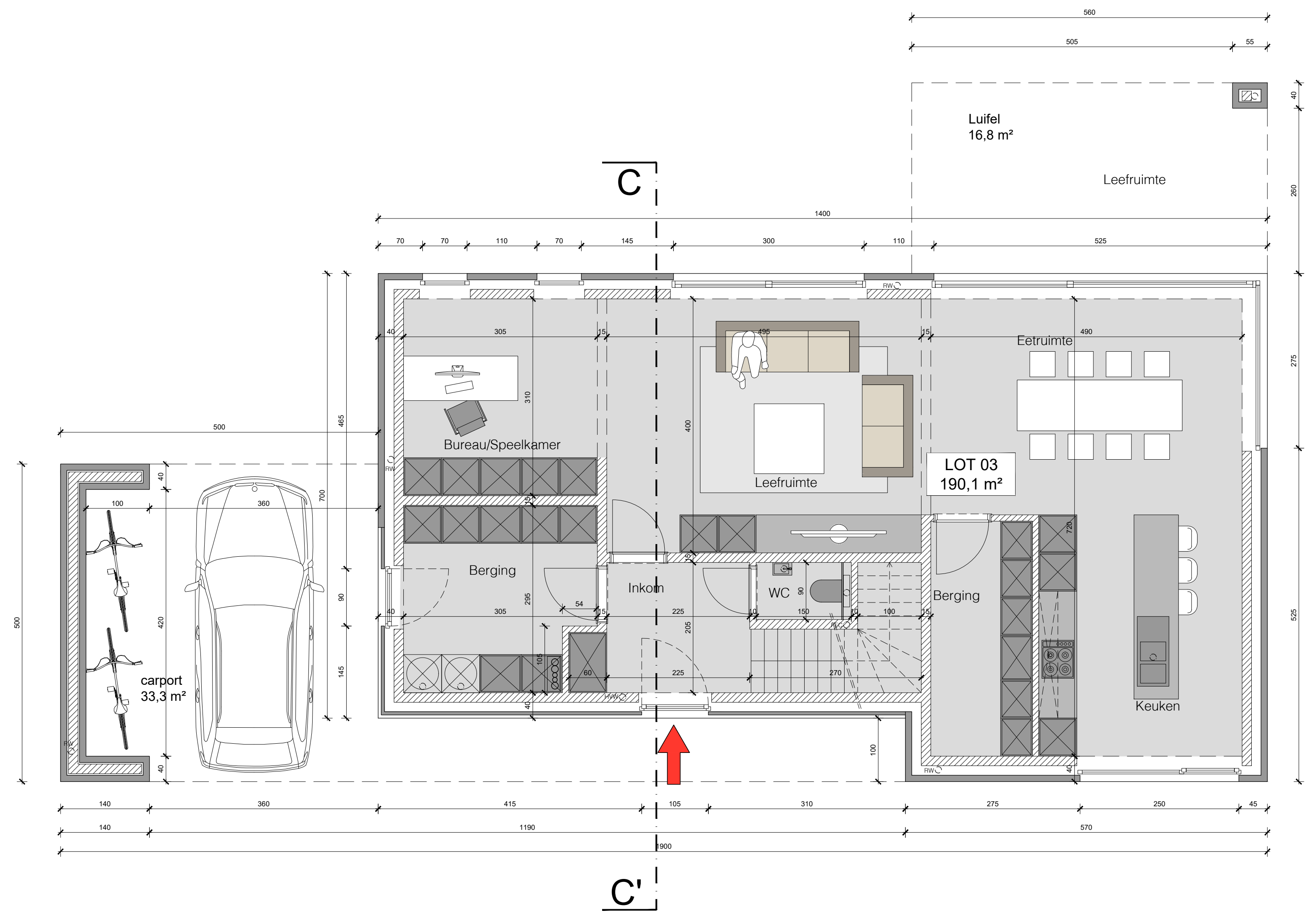
plan GELIJKVLOERS 1/50
